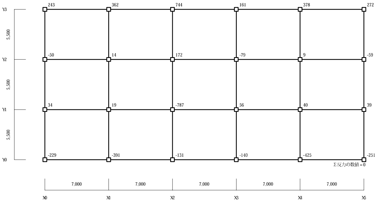
YL加力時/地震荷重時基礎反力図
