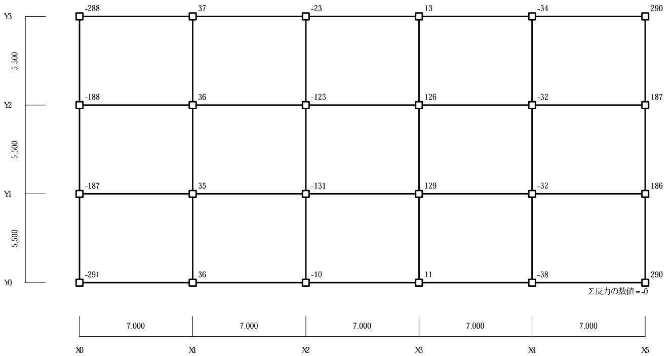
XL加力時/地震荷重時基礎反力図
